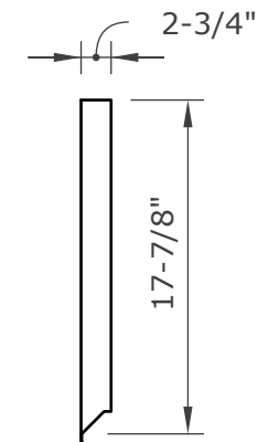
Vent Door - side view
